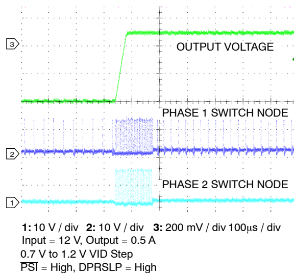
Figure 17. VID Step
