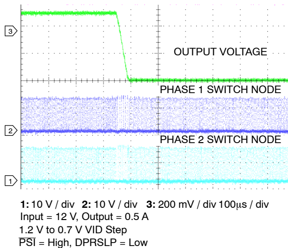
Figure 18. VID Step
