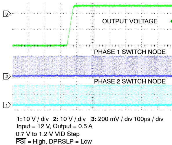
Figure 19. VID Step
