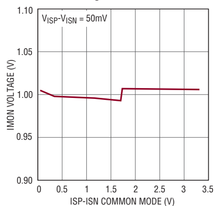
IMON Voltage
