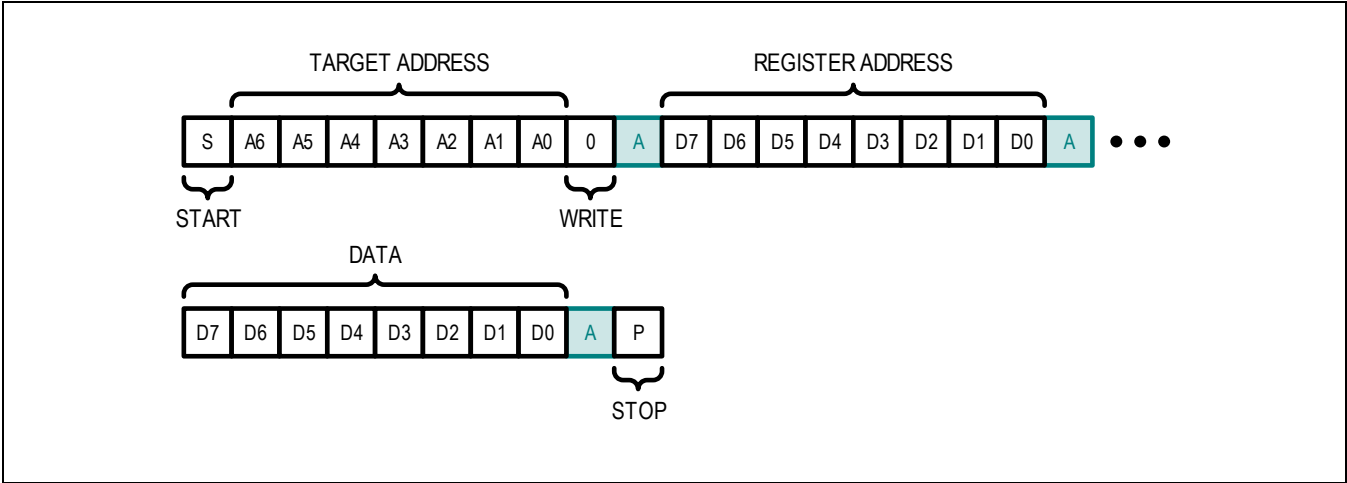
Figure 23. Write Byte
