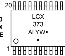
TSSOP-20 DT SUFFIX CASE 948E
