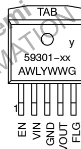
D 2 PAK
