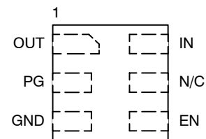
XDFN6
