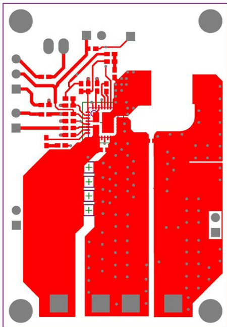
Fig. 20 - Top Layer
