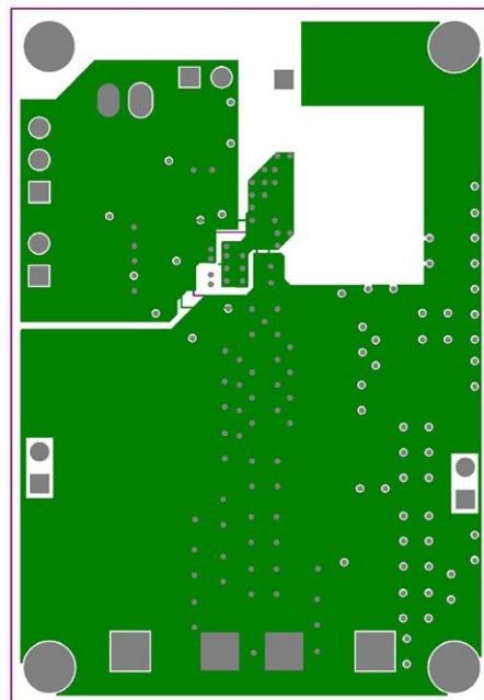
Fig. 22 - Inner Layer 2
