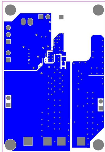
Fig. 23 - Bottom Layer
