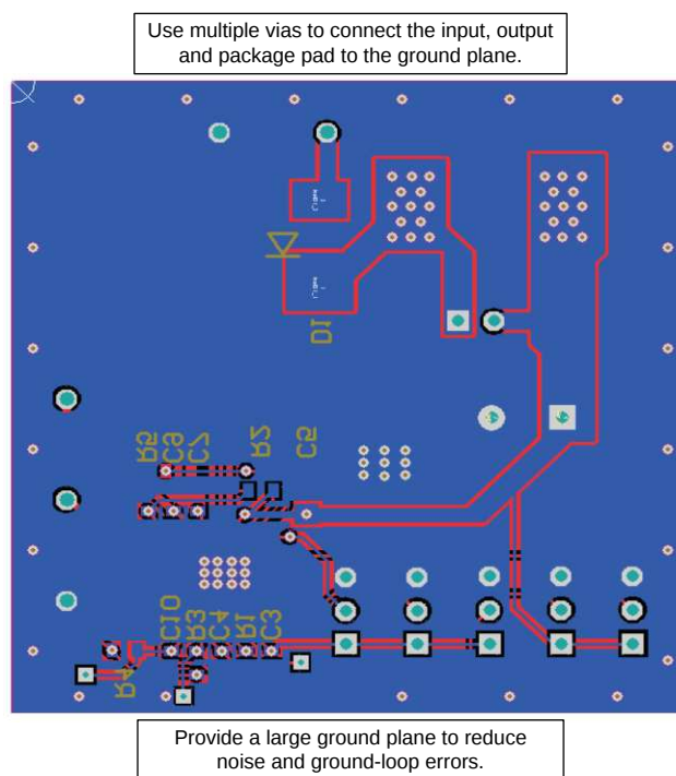
Figure 22. Bottom Layer
