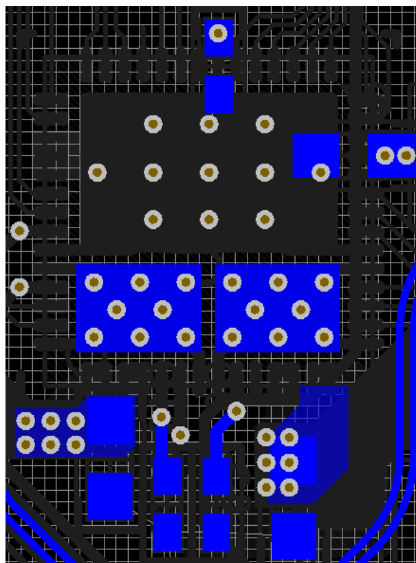
Figure 11-9. Bottom Polygon Pours
