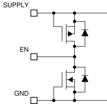
Figure 7-14. EN Pin
