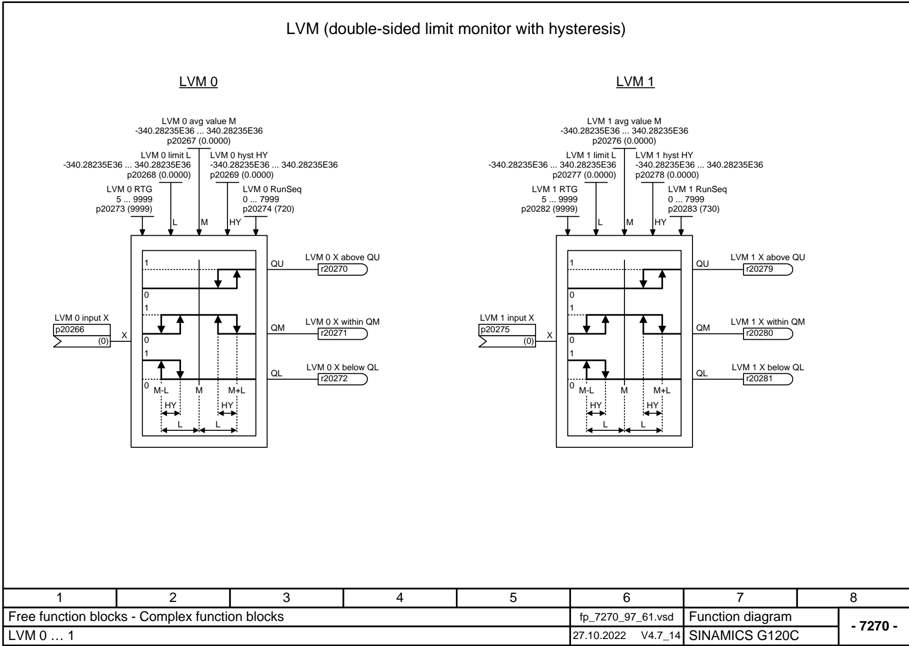
Fig. 3-145 7270 – LVM 0 ... 1
