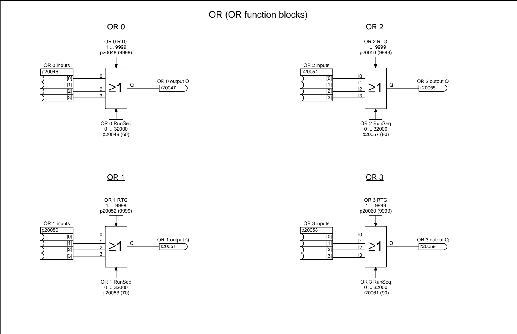
Fig. 3-128 7212 – OR 0 ... 3
