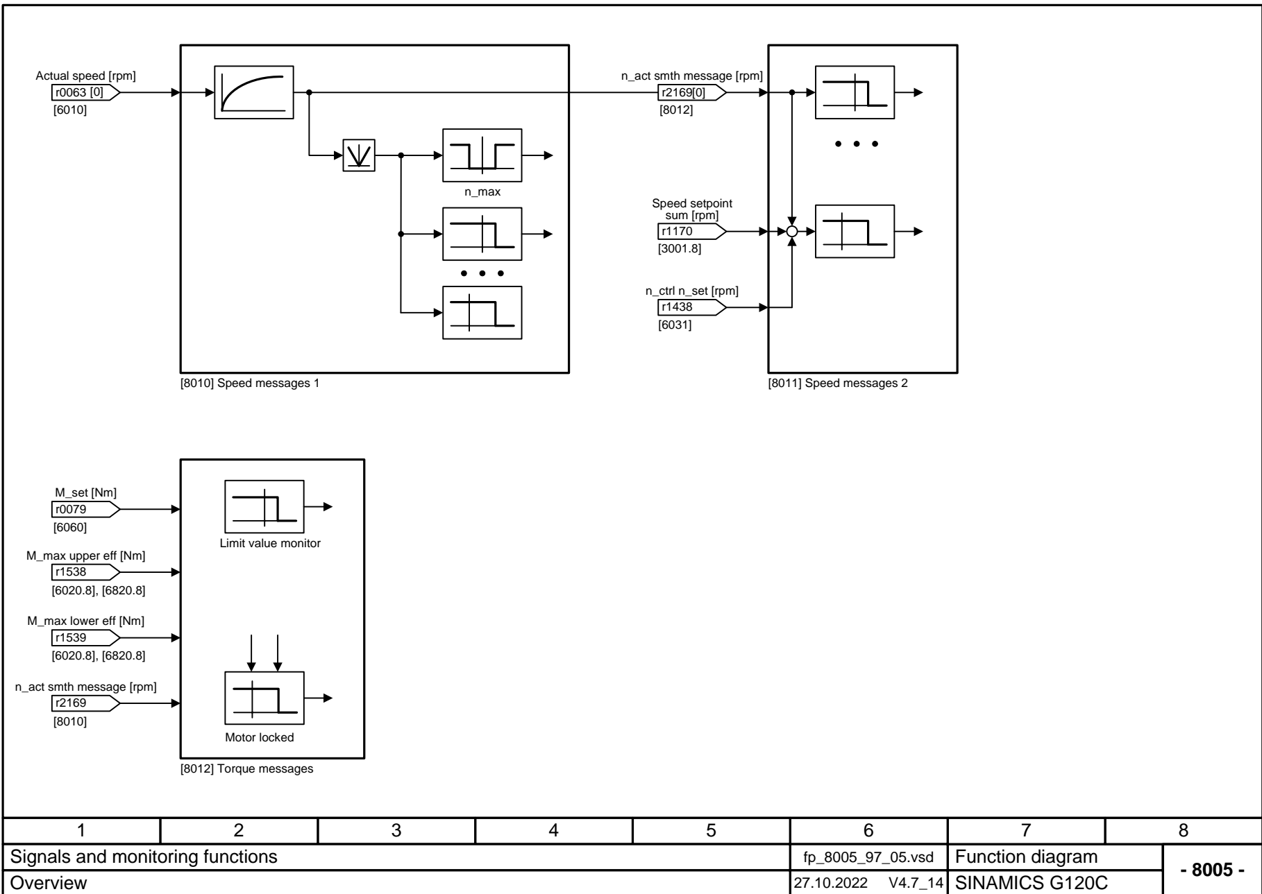
Fig. 3-150 8005 – Overview
