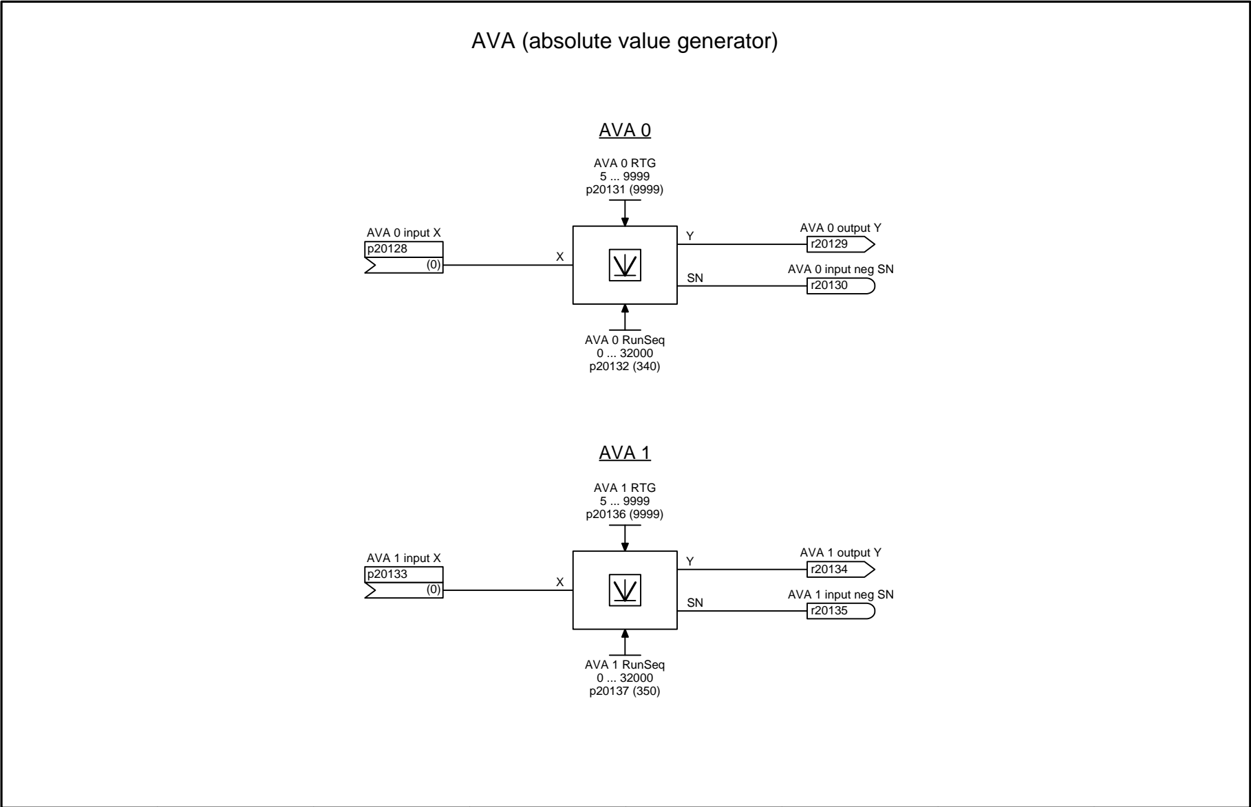
Fig. 3-133 7224 – AVA 0 ... 1
