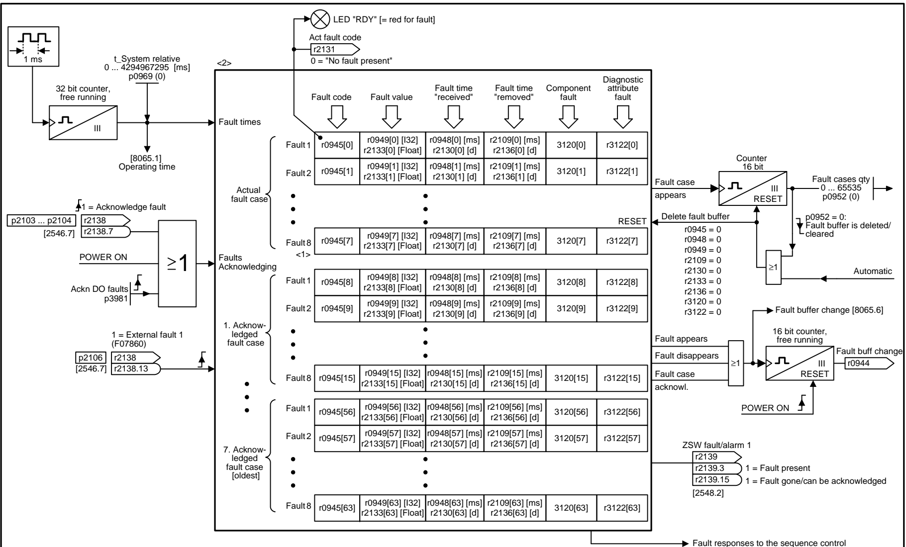
Fig. 3-162 8060 – Fault buffer
