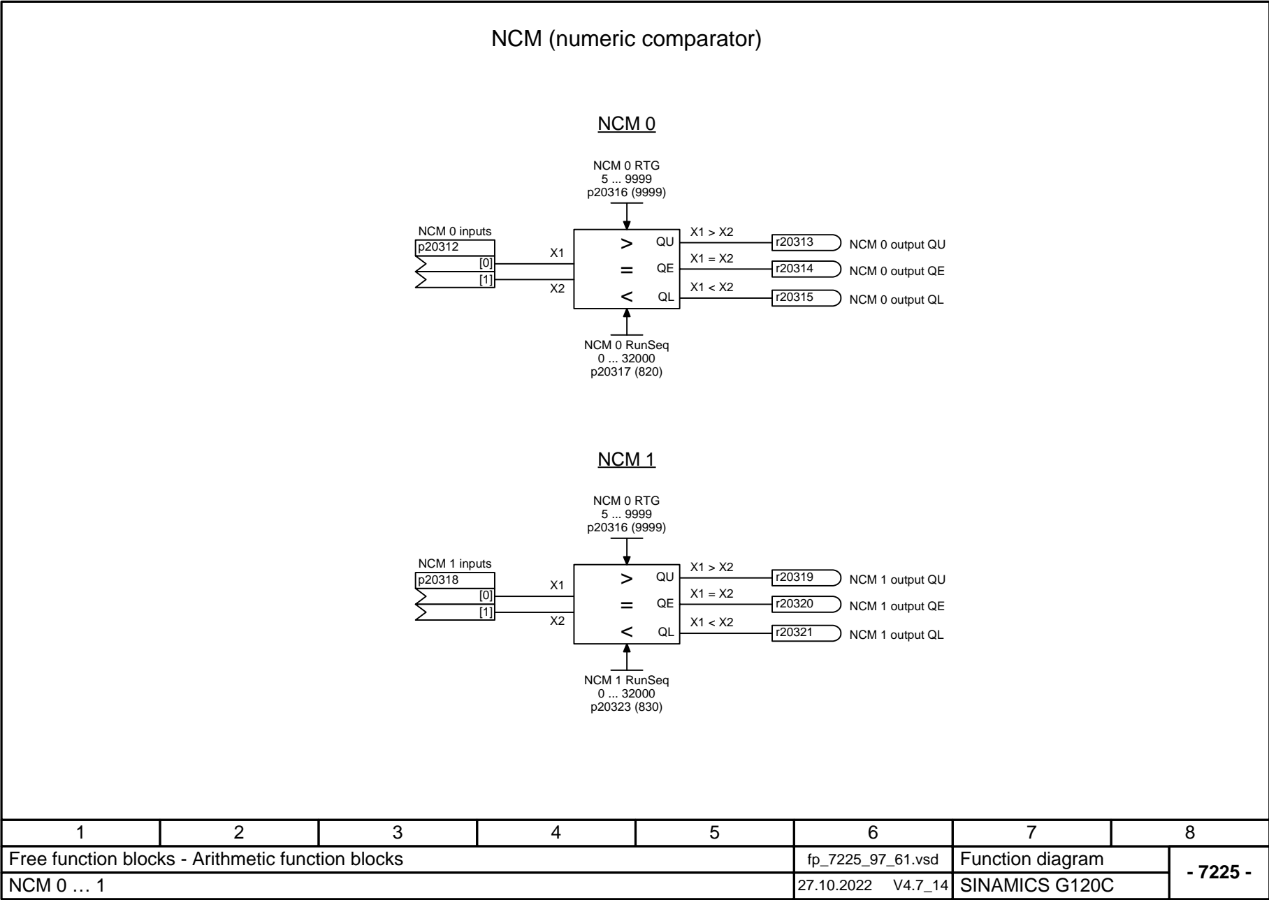
Fig. 3-134 7225 – NCM 0 ... 1
