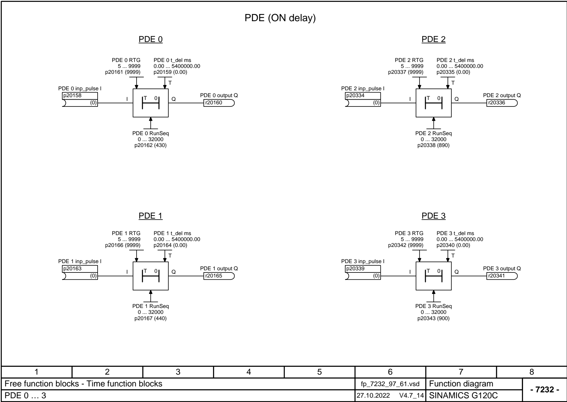
Fig. 3-137 7232 – PDE 0 ... 3
