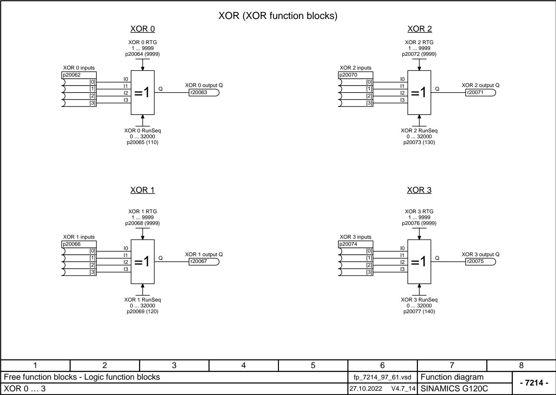
Fig. 3-129 7214 – XOR 0 ... 3
