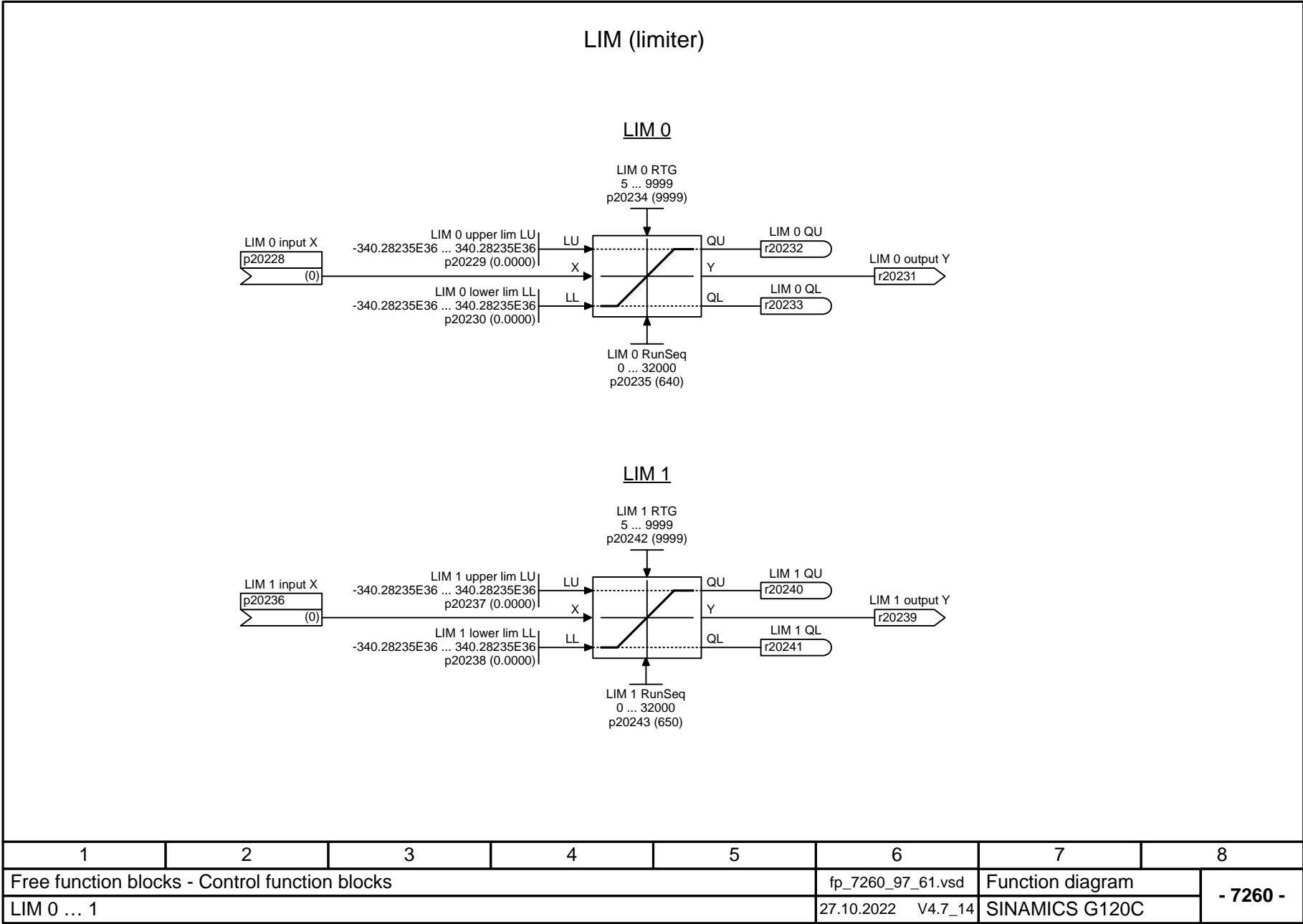
Fig. 3-142 7260 – LIM 0 ... 1
