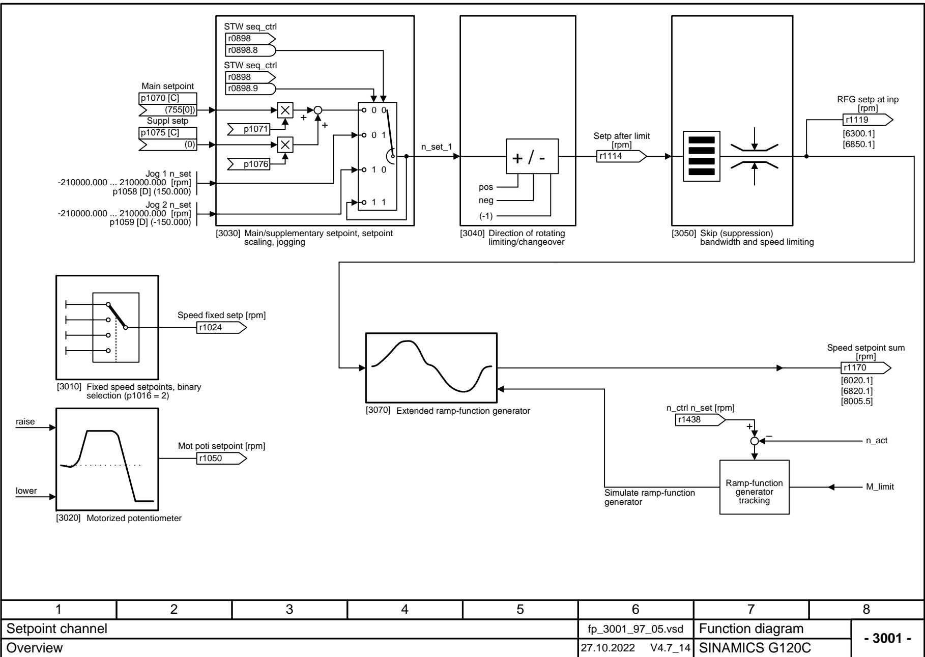
Fig. 3-64 3001 – Overview
