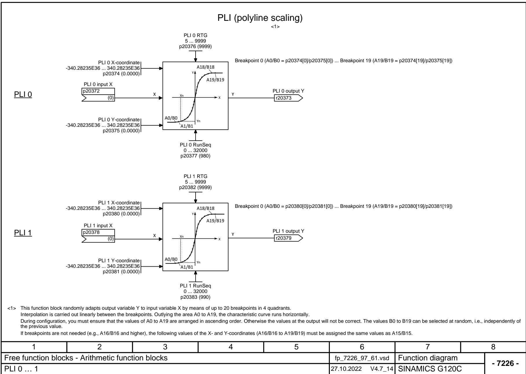
Fig. 3-135 7226 – PLI 0 ... 1
