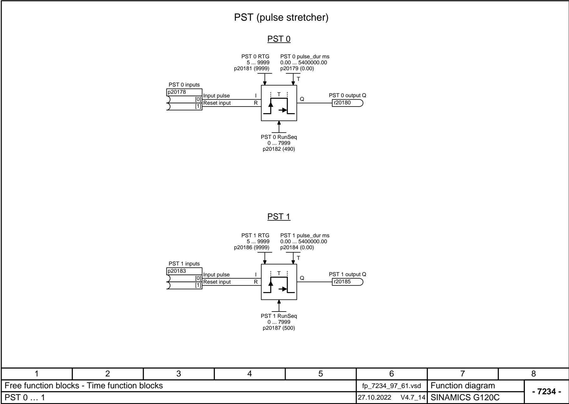
Fig. 3-139 7234 – PST 0 ... 1
