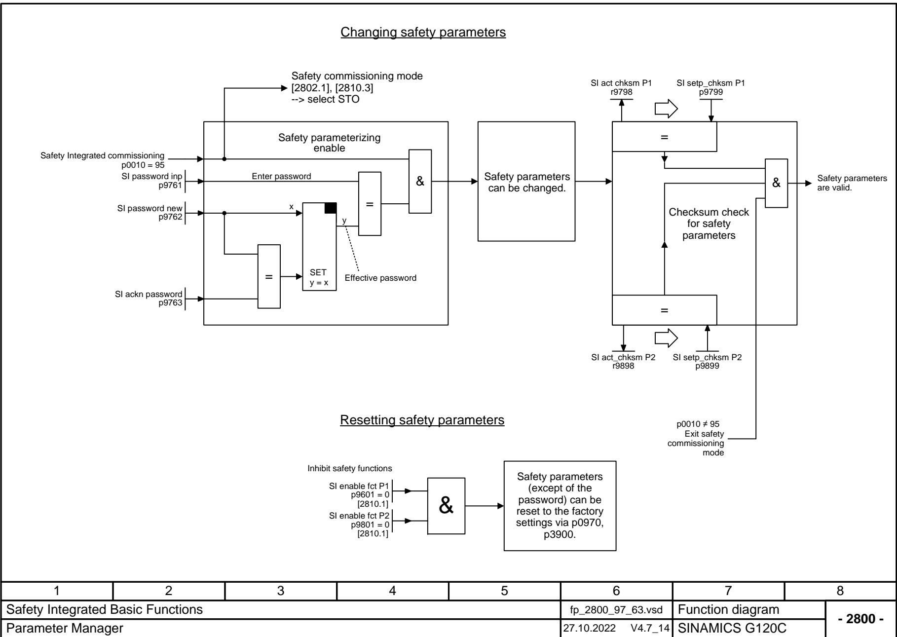
Fig. 3-58 2800 – Parameter manager
