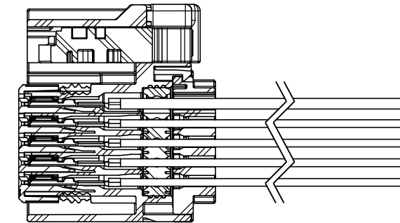
REFERENCE: FRONT RETAINER/SOCKET CONTACT ASSEMBLED STATE フロントリテーナ/ソケット端子装着状態
