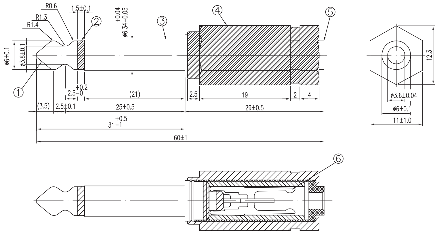
Ø6.3 Mono Plug
