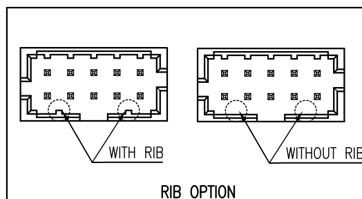
RIB OPTION
