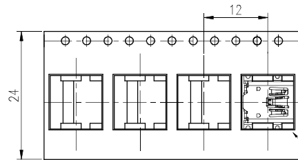
MINI USB B TYPE RECEPTACLE CONNECTOR
