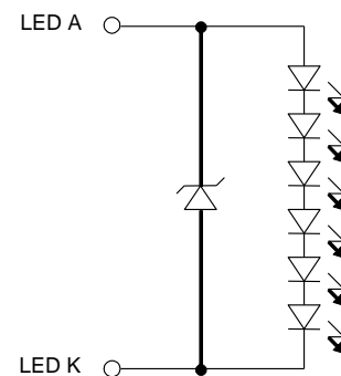
【LED Circuit】
