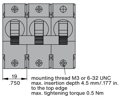
Flange mounting F1 or F4
