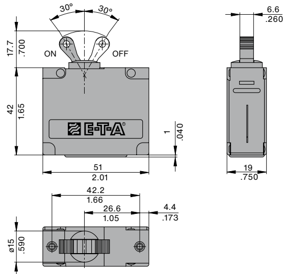
actuator short K, L
