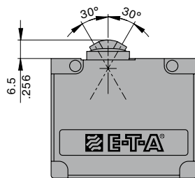
actuator short K, L
