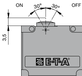
actuator slot Z
