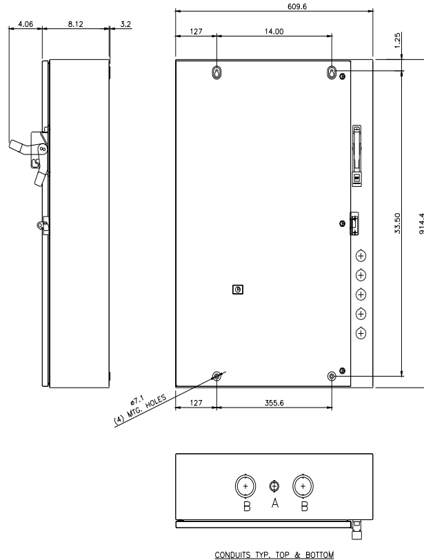
CONDUITS TYP. TOP & BOTTOM
