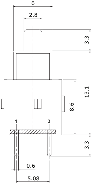
3.3 MM ACTUATOR
