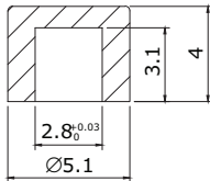
ACTUATOR CAP
