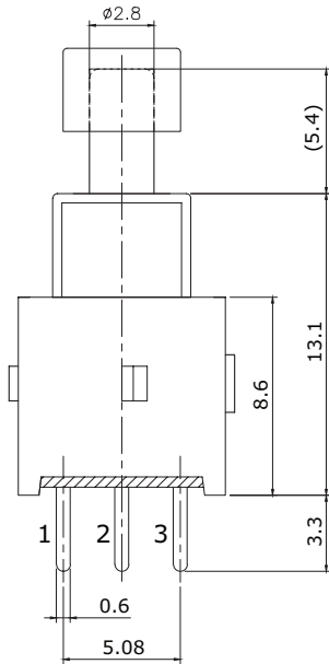
5.4 MM ACTUATOR
