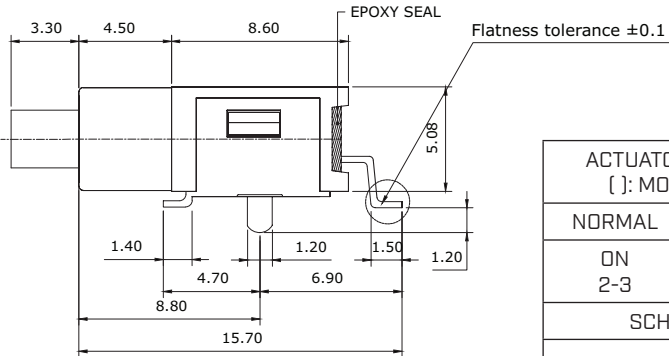
3.3 MM ACTUATOR
