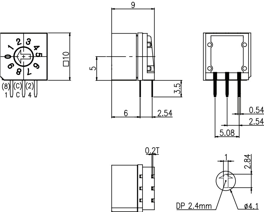
ACTUATOR
