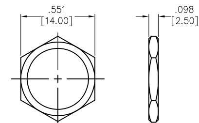
NUT
