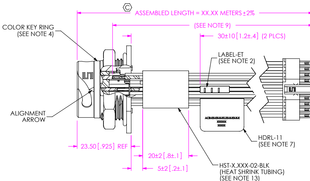
FIG 1 ACR-22-02-X-XX.XX-S-S1-P-1 SHOWN
