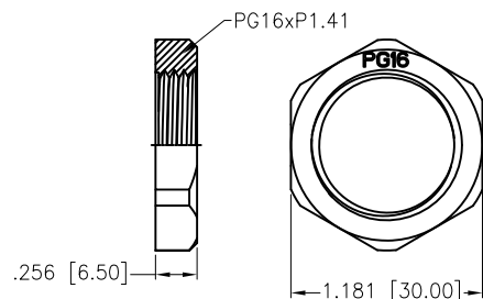
Ⓐ Lock Nut
