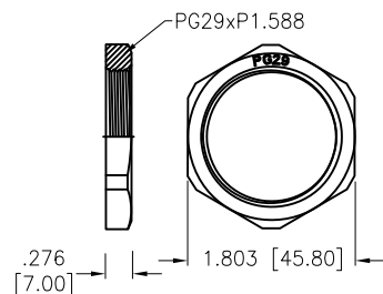
Ⓐ Lock Nut
