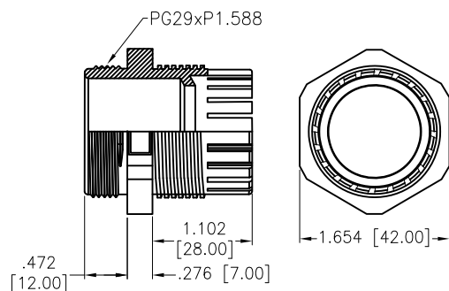
Ⓒ Body
