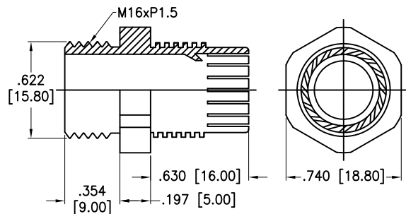
Ⓒ Body
