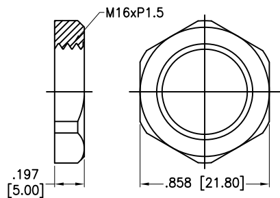
Ⓐ Lock Nut
