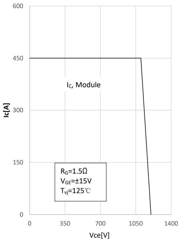
Fig5.RBSOA
