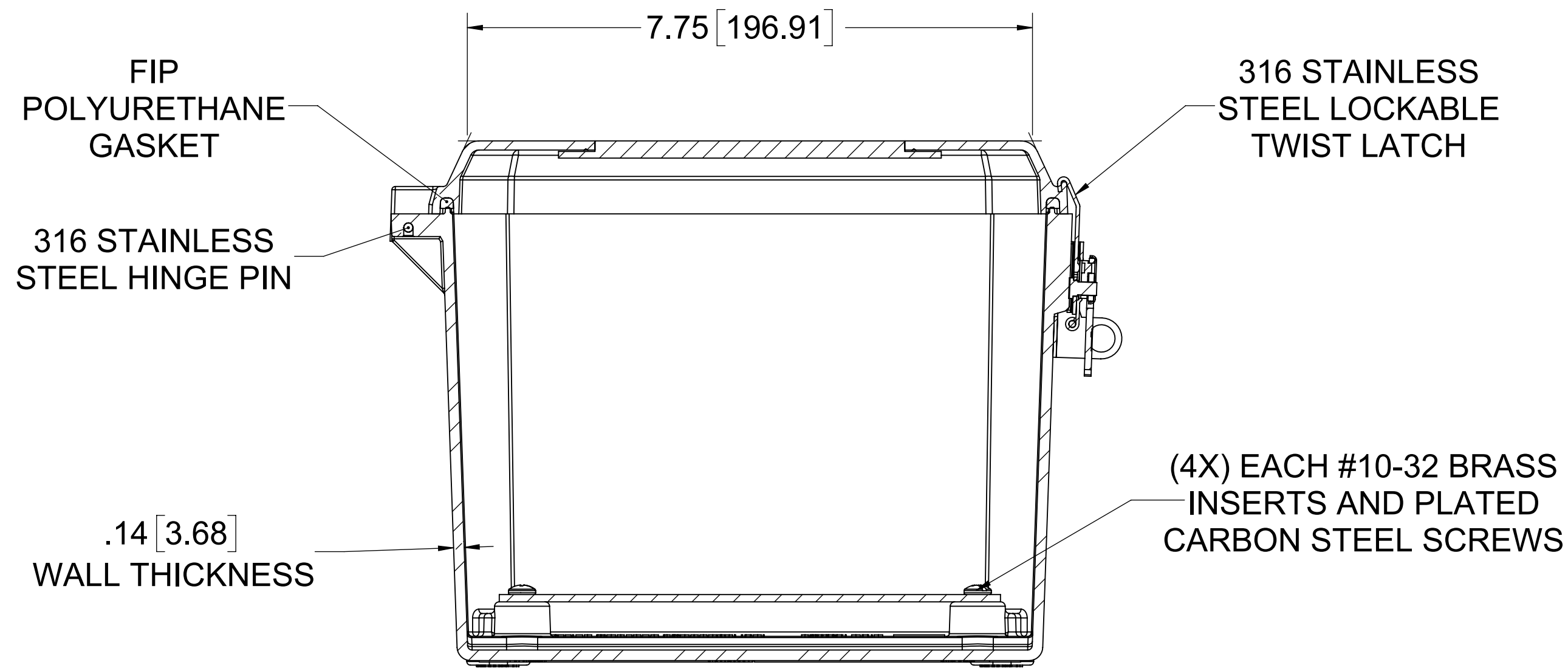
SECTION A-A
