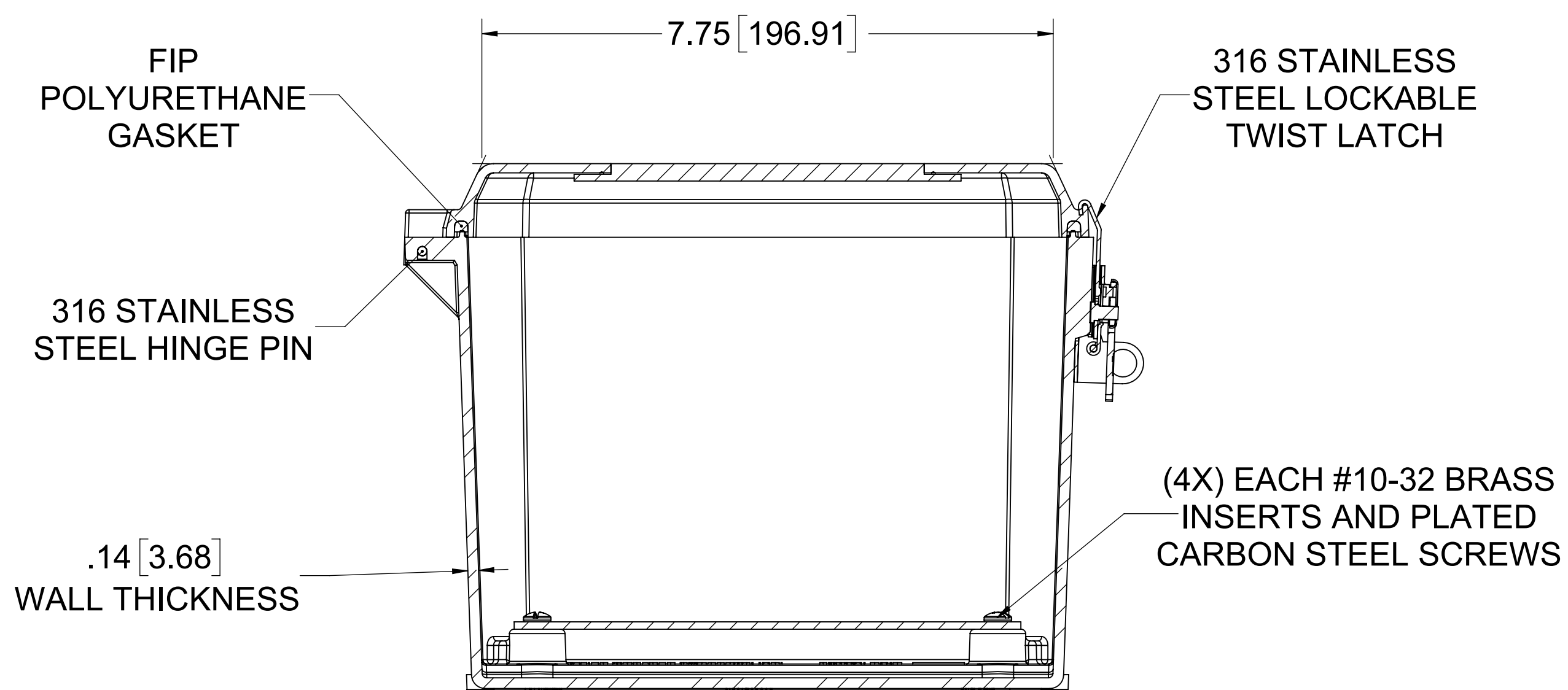
SECTION A-A
