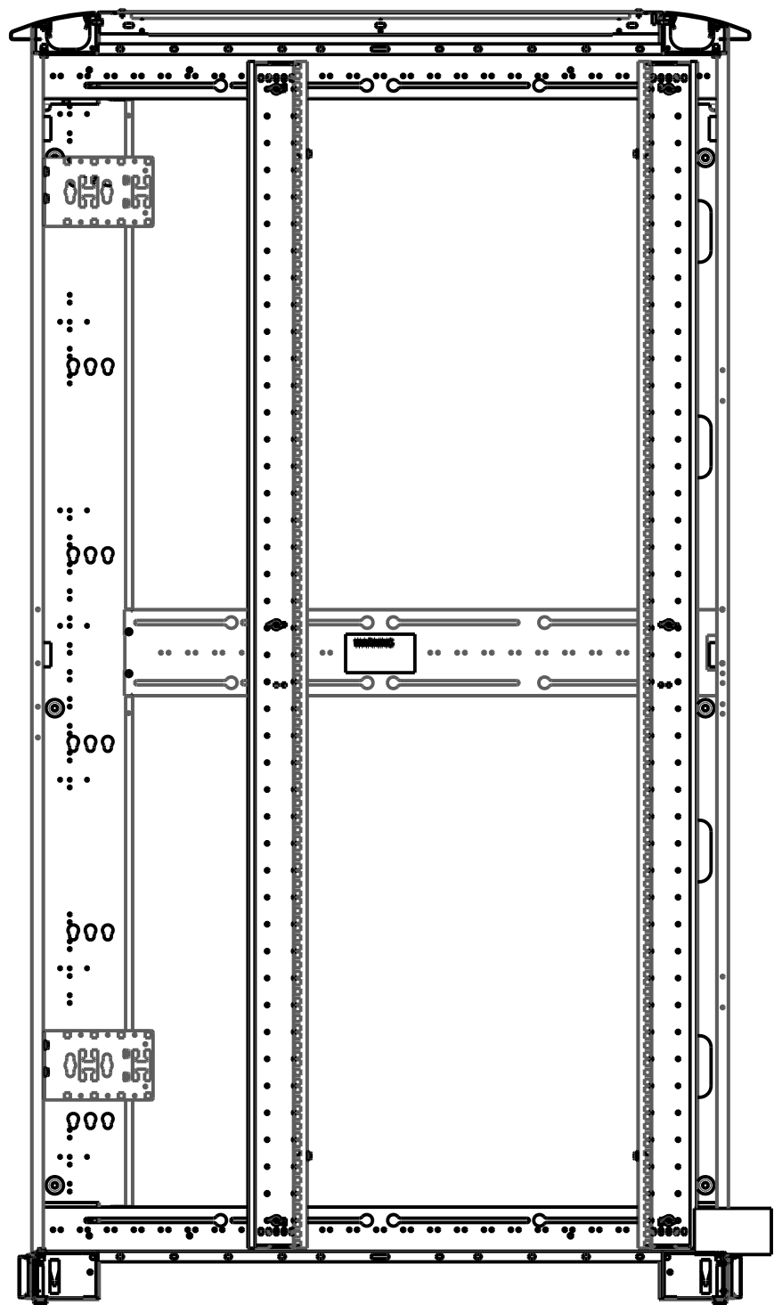
SECTION A-A
