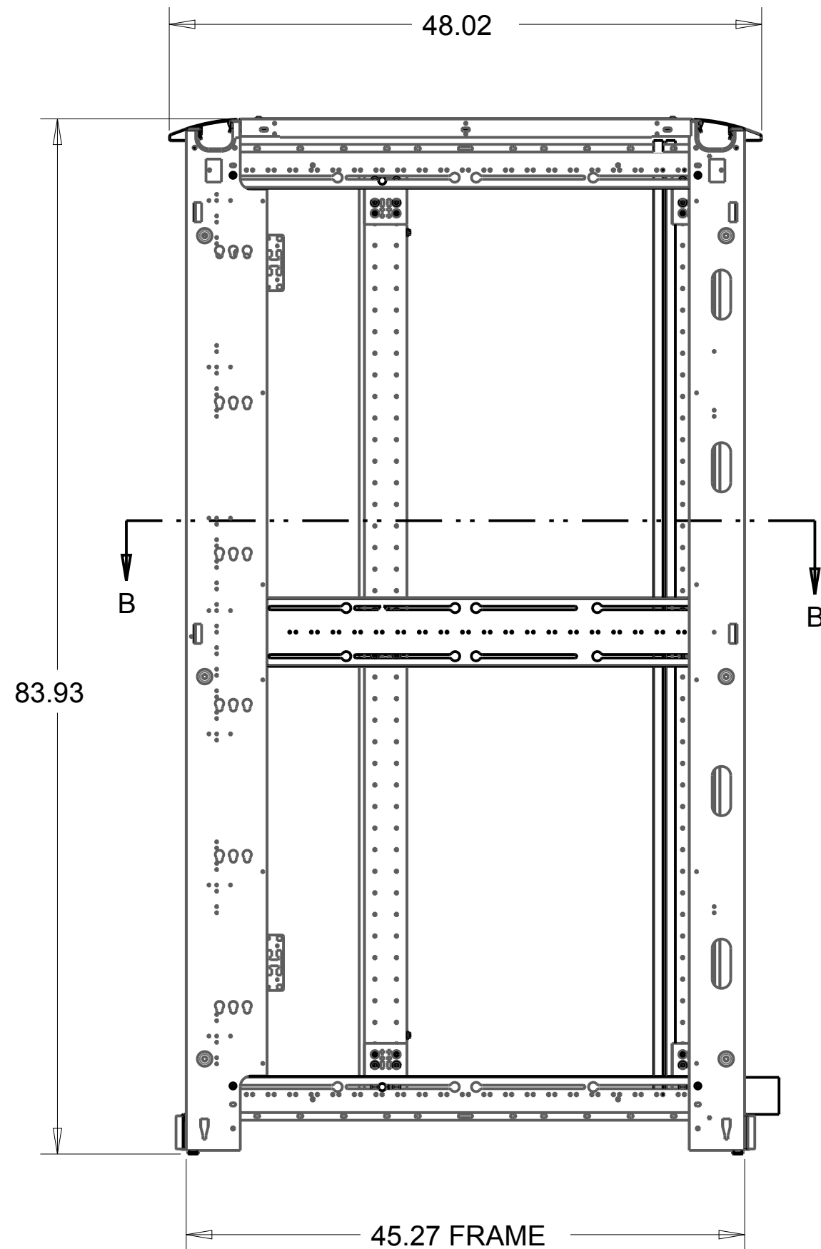
LEFT SIDE
