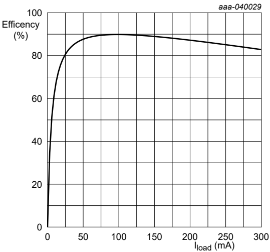
NXF6505B + Wurth 750343725 V_{CC} = 5\text{ V}
