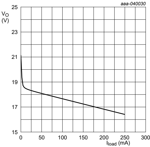
NXF6505B + Wurth 78931812518 V_{CC} = 5\text{ V}
