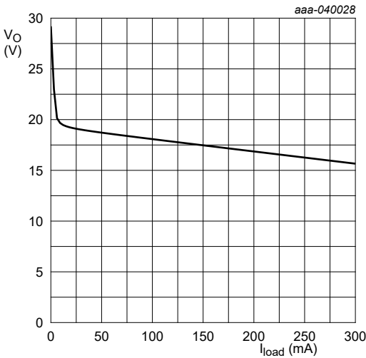
NXF6505B + Wurth 750343725 V_{CC} = 5\text{ V}
