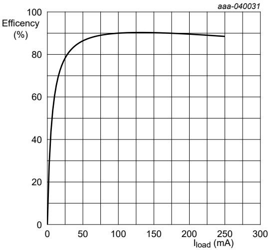
NXF6505B + Wurth 78931812518 V_{CC} = 5\text{ V}
