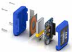
STEVAL-MKBOXPRO
