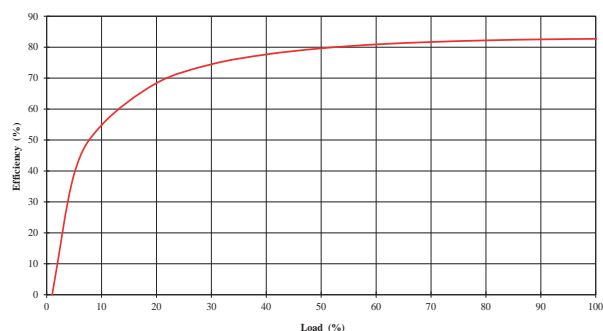
NMK0505TSAC
