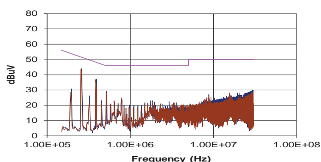
NMK0505TSAC (Average)
