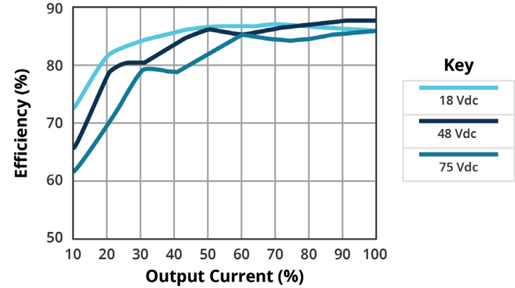
EFFICIENCY VS OUTPUT LOAD PDQ15-Q48-D15-D
