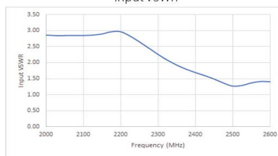
Input VSWR
