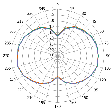
XZ-Plane Gain
