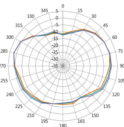
YZ-Plane Gain
