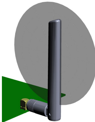
YZ-Plane Gain
