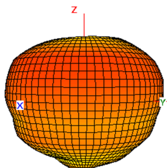
2450 MHz
