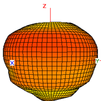
2400 MHz
