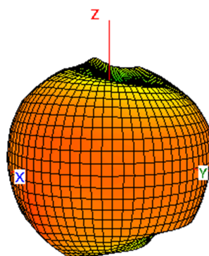
2450 MHz
