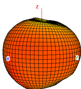
2400 MHz
