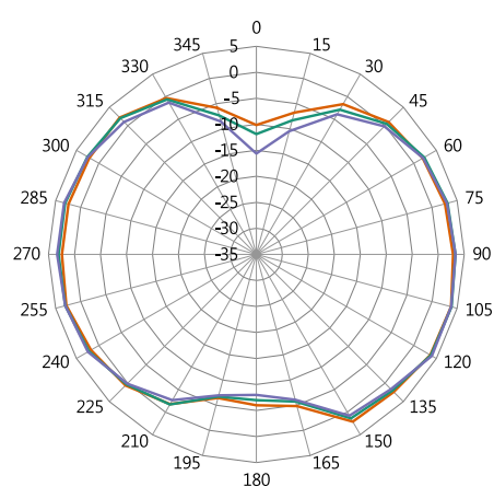
2400 MHz
