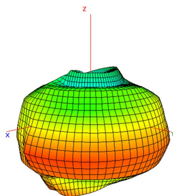
778 MHz
