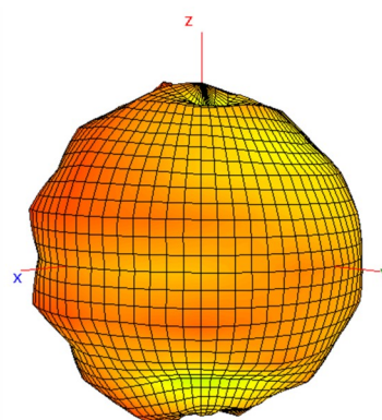
778 MHz
