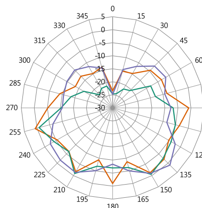
YZ-Plane Gain
