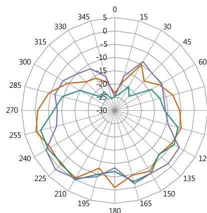
XZ-Plane Gain
