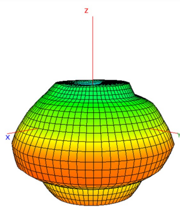
778 MHz
