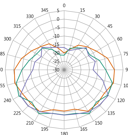
YZ-Plane Gain
