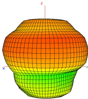
5150 MHz
