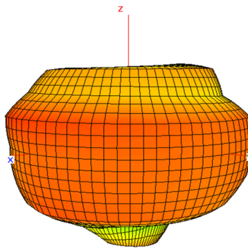
3355 MHz
