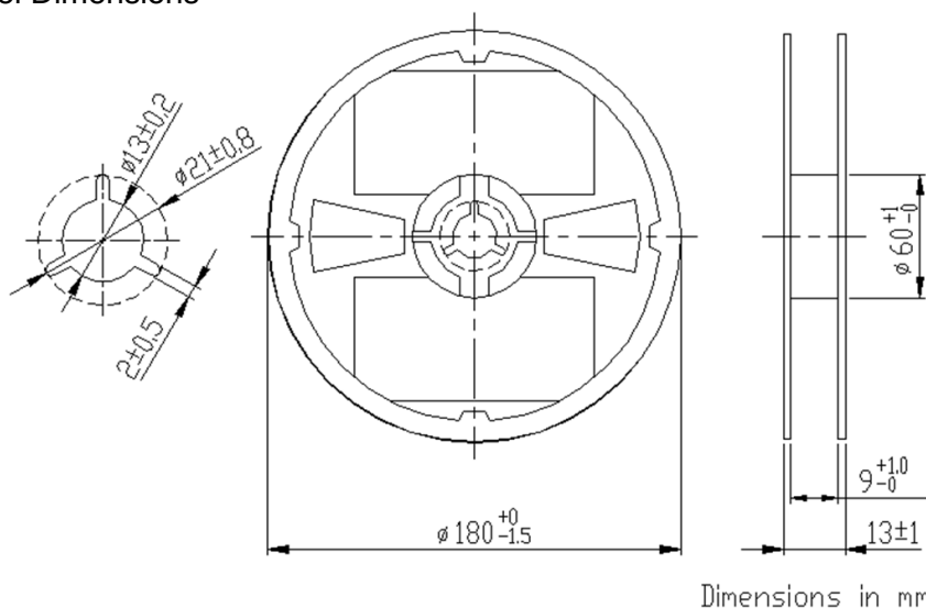
Reel Dimensions
