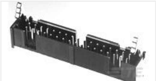
TE Part #1761608-5 IDC LOW PRO HDR 14P VERT SHT L
