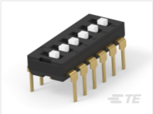
TE Part #2454982-4 ADE Next Gen. 06 Pos. THT TU
