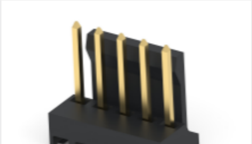
TE Part #3-1744163-5 05P MTA100 HDR ASSY SM 30AU LF T&R
