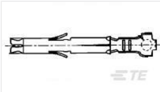
TE Part #170365-3 MINI UNIVERSAL M-N-L SOCKET LP
