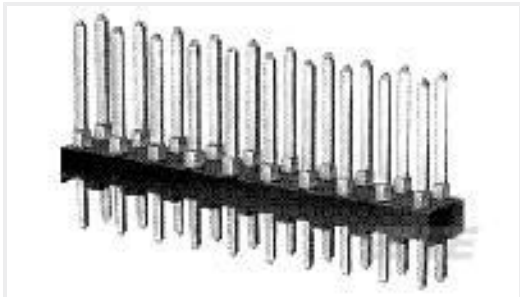
TE Part #1-87227-2 24 MODII HDR DRST UNSHRD .100
