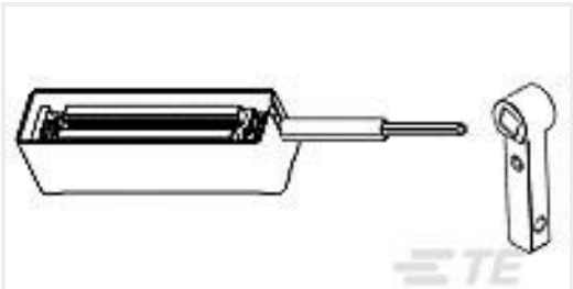
TE Part #6674720-1 TC ZIF REC ASSEMBLY,KIT INV.
