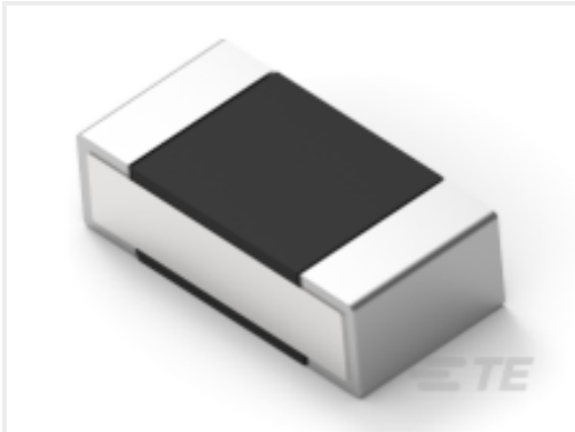
TE Part #2176308-4 RP 1E 0.1W 143K 0.1% 25PPM 5K RL
